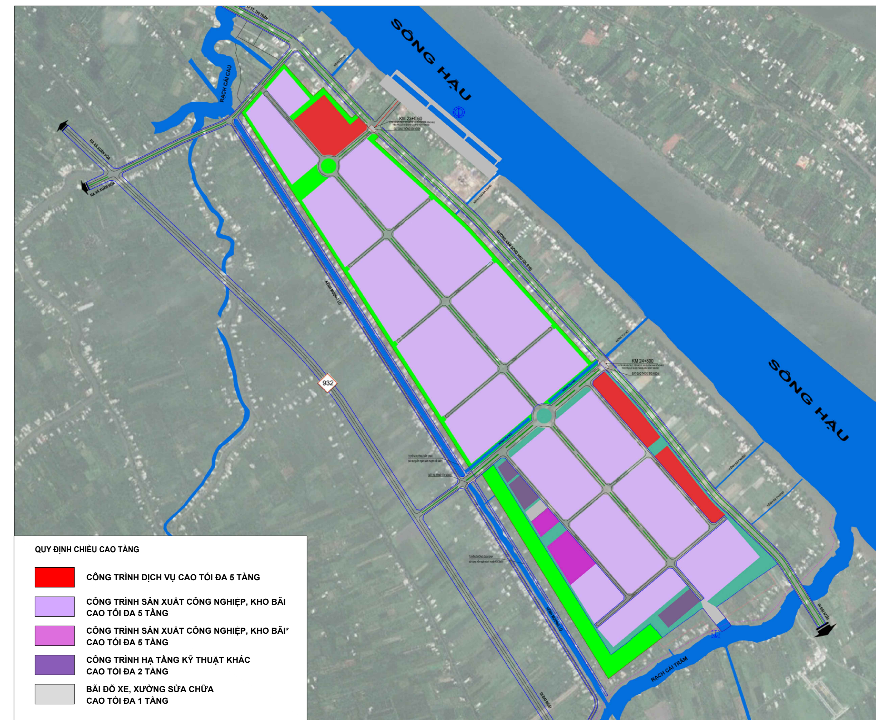
SƠ ĐỒ KHÔNG CHẾ CHIỀU CAO TẦNG CÁC CÔNG TRÌNH
