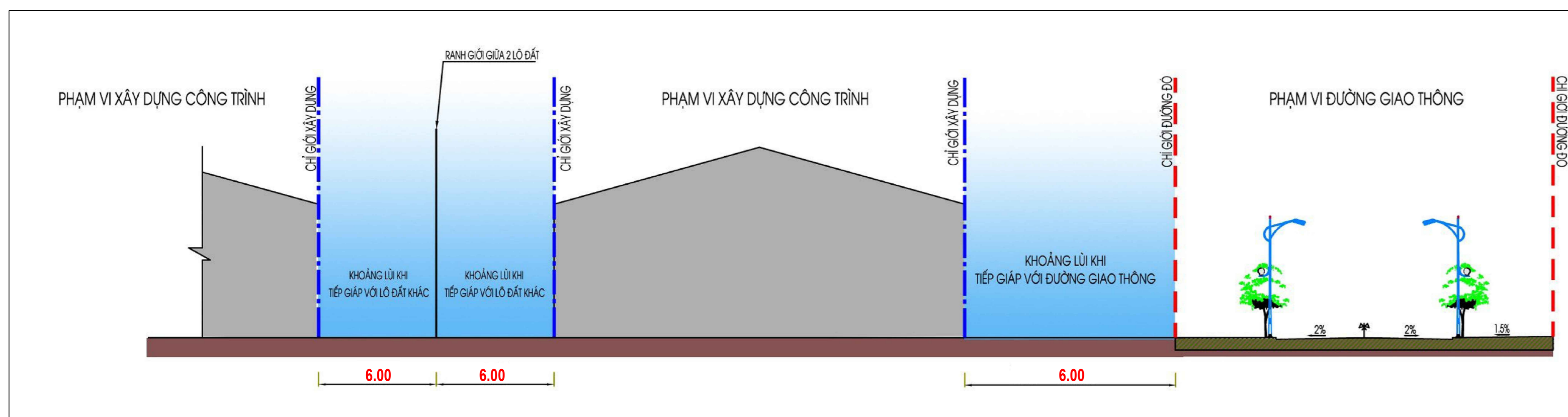
KHÔNG CHẾ KHOẢNG LỬI XÂY DỰNG CÔNG TRÌNH VỚI CHỖ GIỚI ĐƯỜNG ĐỎ VÀ VỚI CÔNG TRÌNH LÂN CẬN
